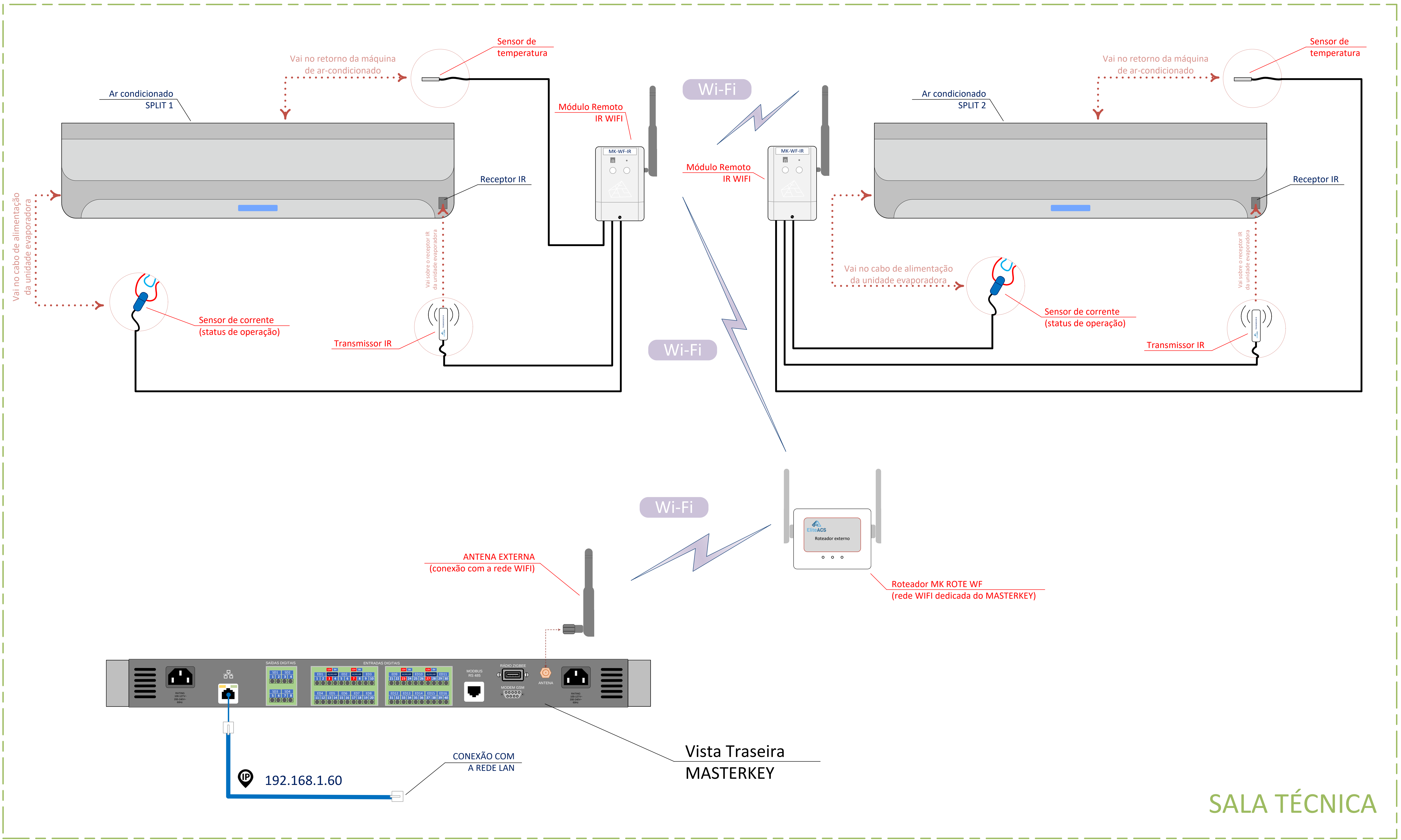
1 Esquema de ligação orientativo Automação de equipamentos de ar-condicionado
